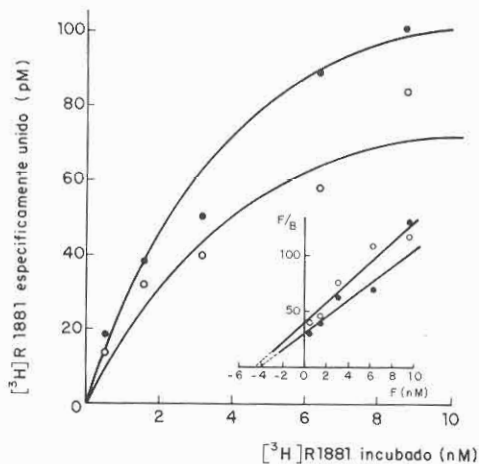
FIG. 2 - Curva de saturação do andrôgeno sintético [^3\text{H}]\text{R1881} especificamente unido à fração citosólica de homogeneizados de próstatas de ratos controle (o—o) e tratados com dose farmacológica de extrato de S. rebaudiana . O inserto mostra o gráfico de Eadie-Hofstee ("inversão de Wilkinson") para determinação da quantidade total de sítios receptores (Q) e da constante de afinidade aparente ( K_a ) do complexo H-R, segundo a equação F/B = F/Q + Q/K_a (Rodbard & Feldman, 1975). Abreviaturas: F (free = hormônio livre; B (bound) = hormônio unido.
